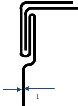
Figura 3: Unión longitudinal
